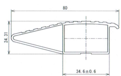
アルミステップ断面図 S=1:1
