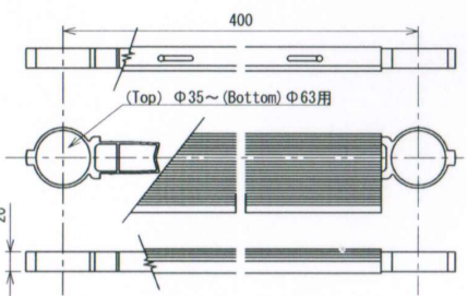
アルミステップ側面図 S=1:5
