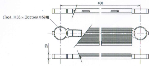
アルミステップ側面図 S=1:5
