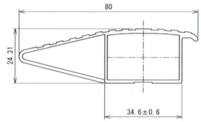
アルミステップ断面図 S=1:1
