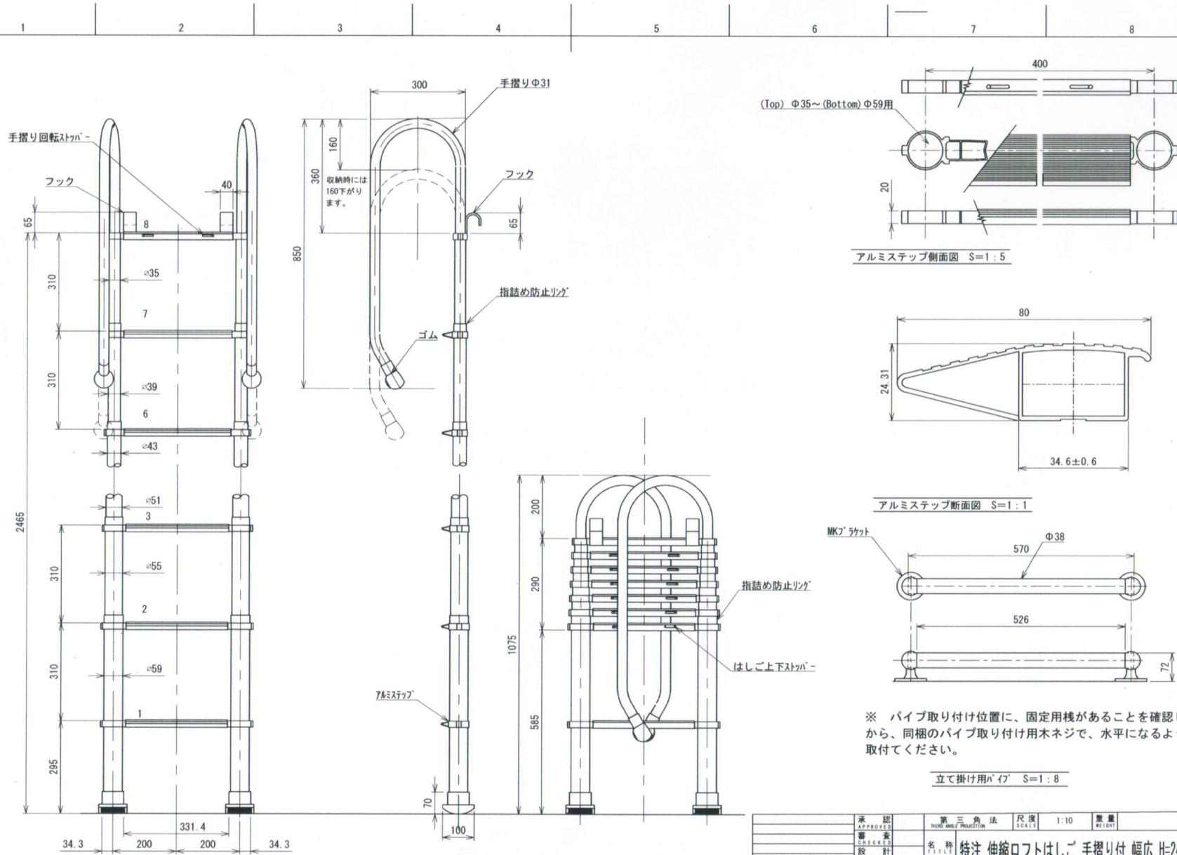
使用時側面図 収納時手摺り収まり
